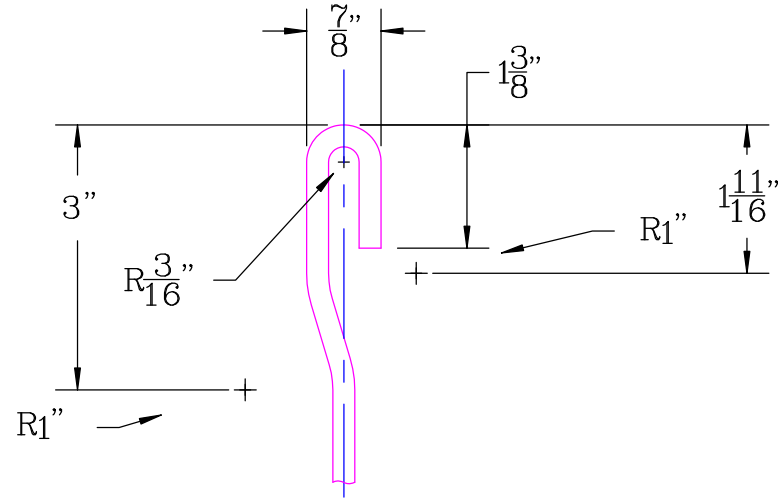
VIEW A-A
